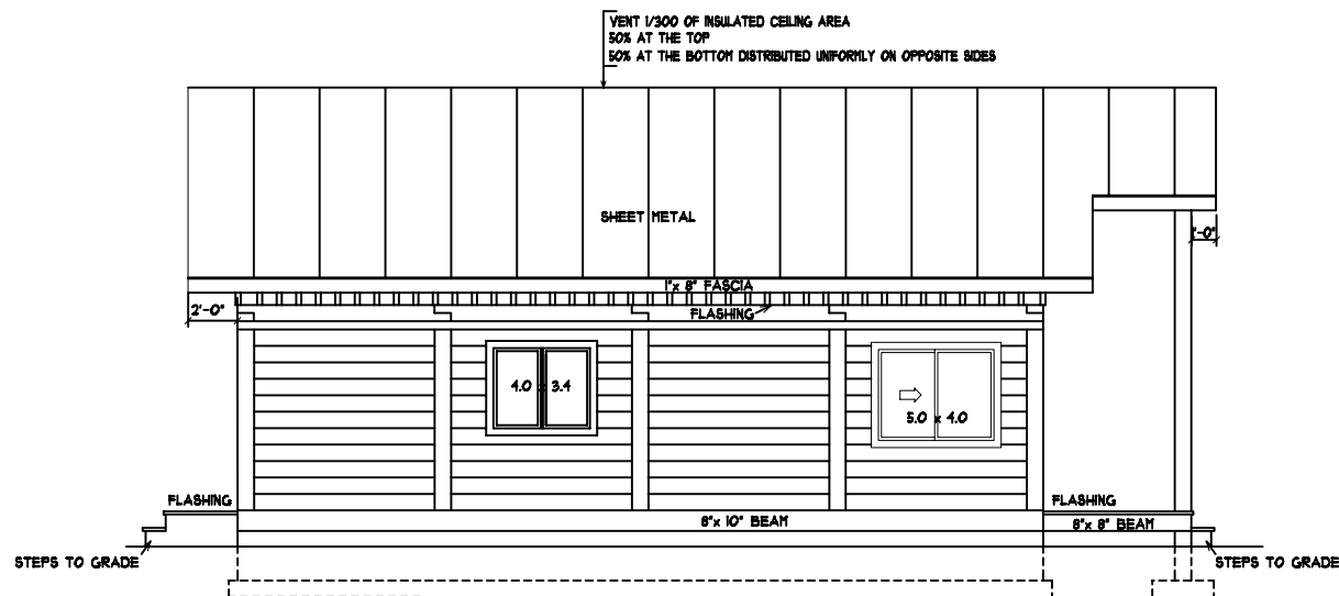
RIGHT ELEVATION
